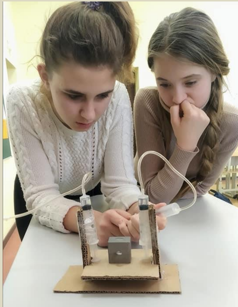
Створення механізму «Гідравлічний ліфт»
